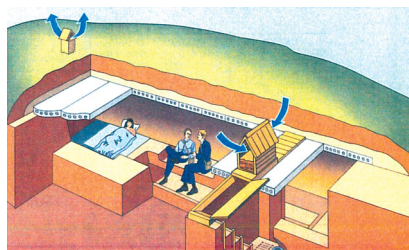
Быстровозводимое противорадиационное укрытие из железобетонных плит
